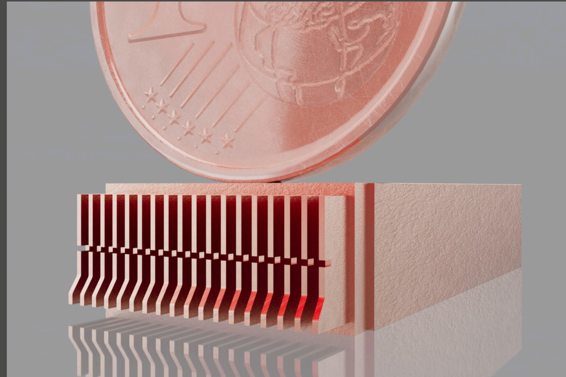
Kupferelektrode, Schlitzbreite 0,2 mm, Stegbreite 0,1 mm \triangleq Formkontur Schlitz 0,12 mm, Steg 0,18 mm, Oberfläche VDI
